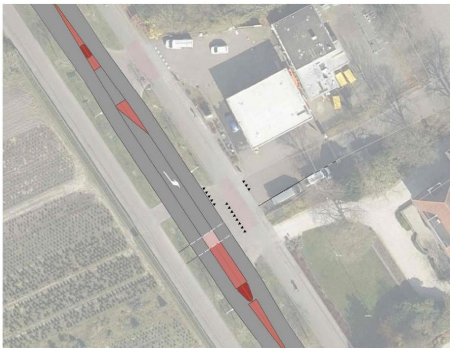
Figuur 12 Schetsontwerp voorsorteerstrook Rijksstraatweg/Esseberg
