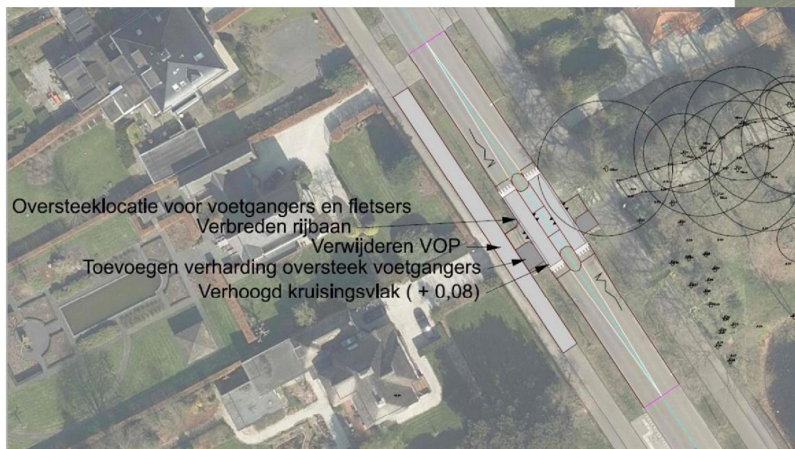
Figuur 17 grove schets aansluiting landgoedlaan Rijksstraatweg landgoedlaan variant a & b
